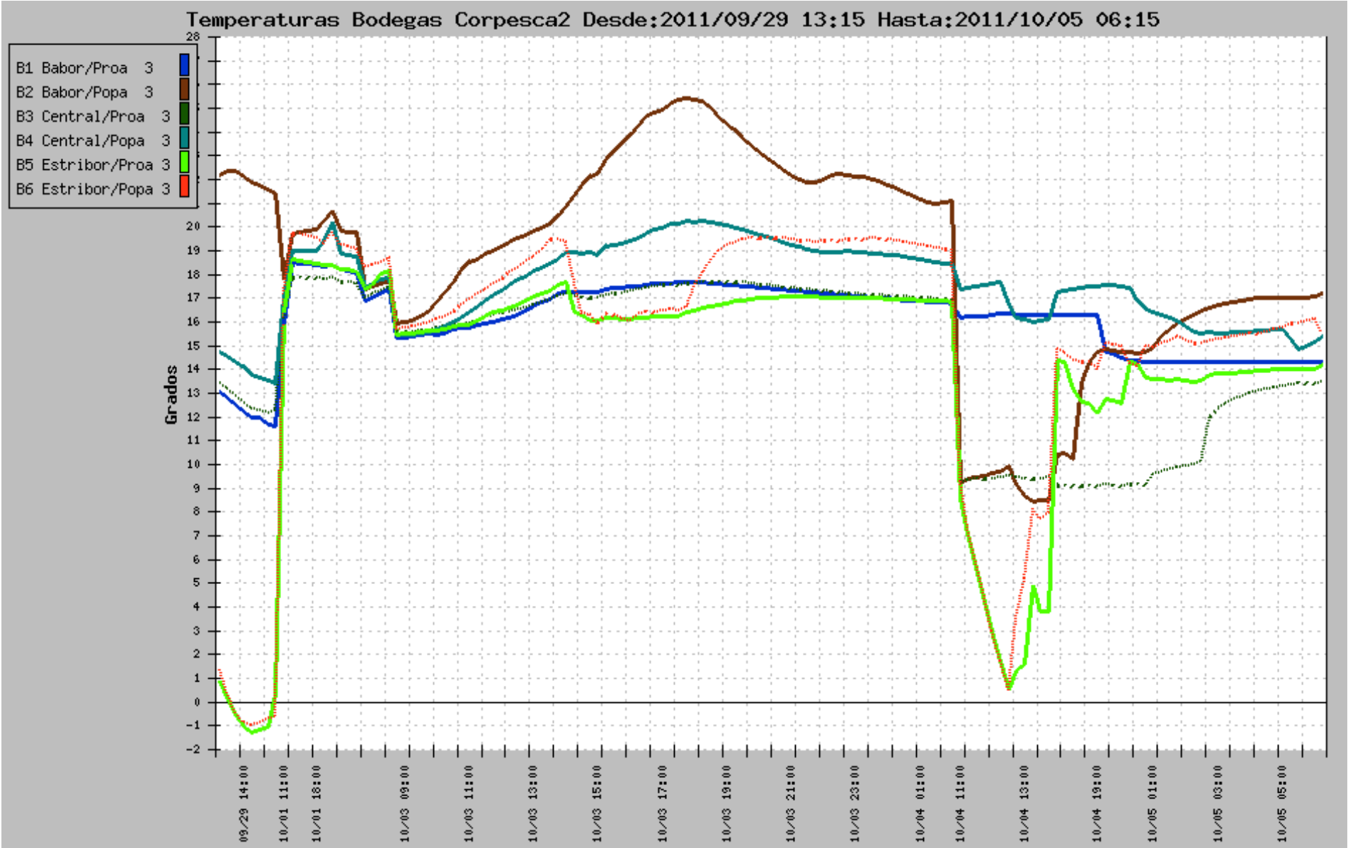
Corpesca S.A. Grafico Sala Control Temperaturas de Bodega Corpesca2.
